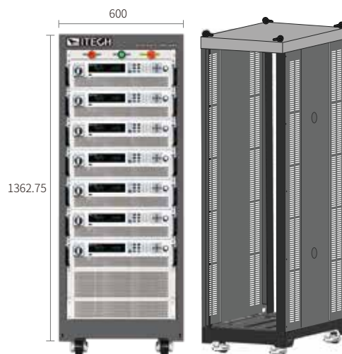
IT-E4029-27U (尺寸单位: mm)
